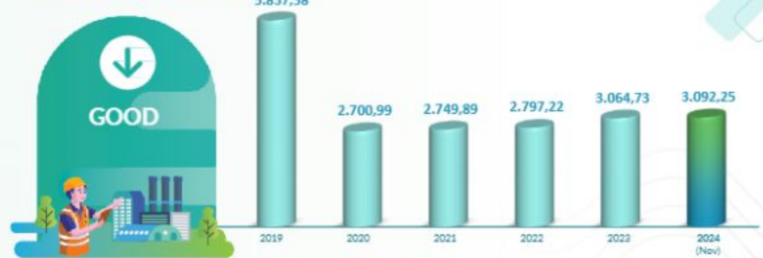
NPHR (kcal/kwh)
